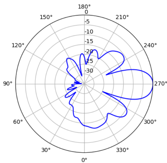
5GHz (Vertical)
