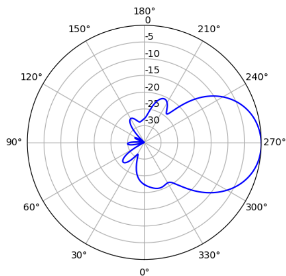
2.4GHz (Vertical)
